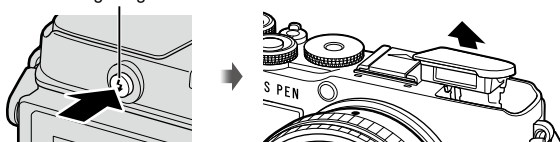
Blitzentriegelungstaste
