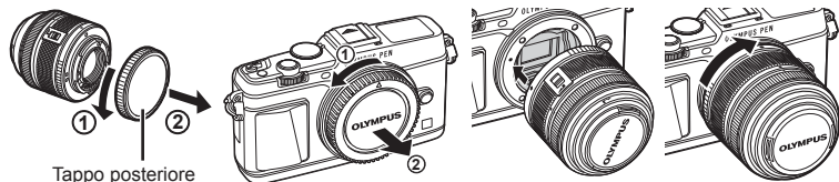
Tappo posteriore
